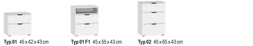
Typ 01 45 x 42 x 43 cm Typ 01 F1 45 x 55 x 43 cm Typ 02 45 x 65 x 43 cm
